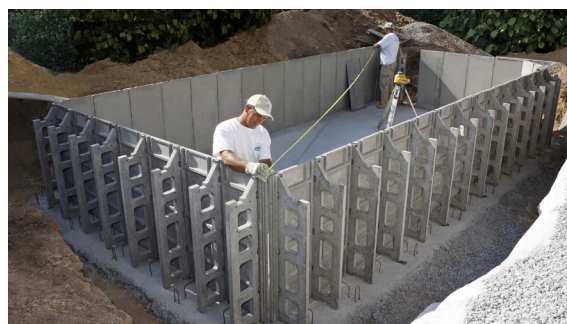
4 - Fixation et réglage des panneaux modulaires
